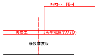
施工要領図
